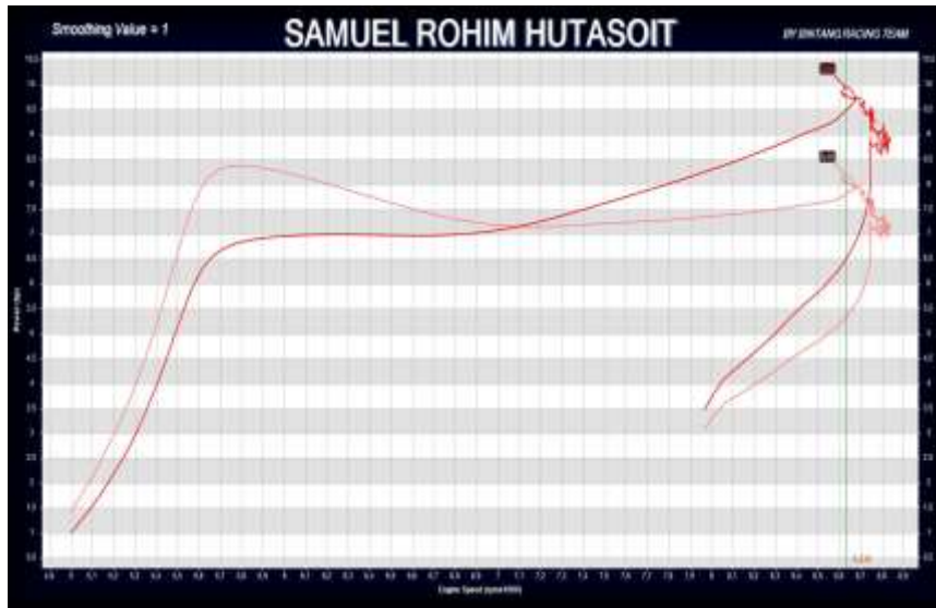
Gambar 4.1 Grafik pulley standar (Sumber : dokumen penelitian)
